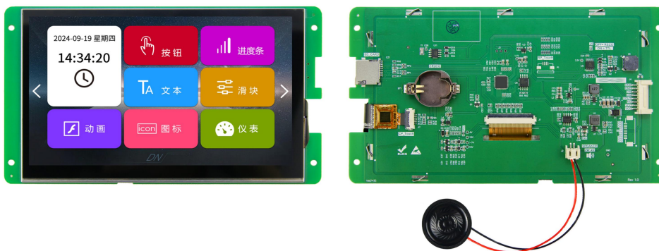
图 1-2 7.0 寸电容触摸参考图
