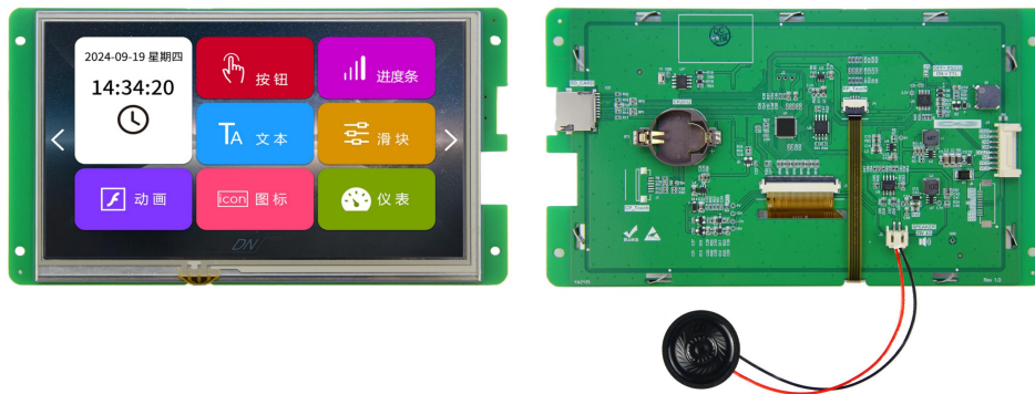
图 1-1 7.0 寸电阻触摸参考图
