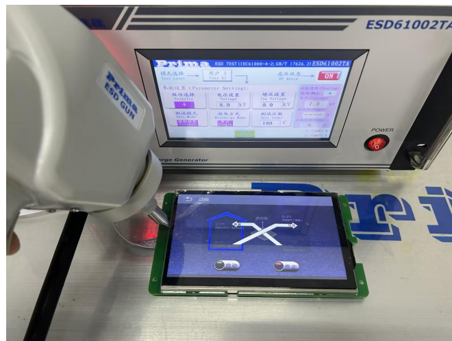
图 4-2 ESD 测试图
