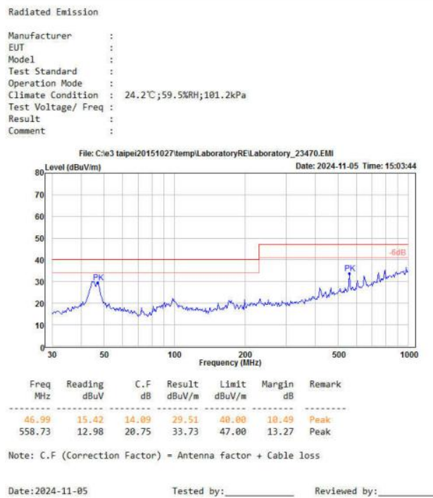
图 4-6 RE 测试垂直方向
